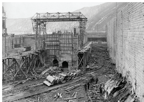
Stavba vorové plavební komory. Tunely v dělicí zdi přivádějí a odvádějí vodu Archiv Povodí Vltavy
