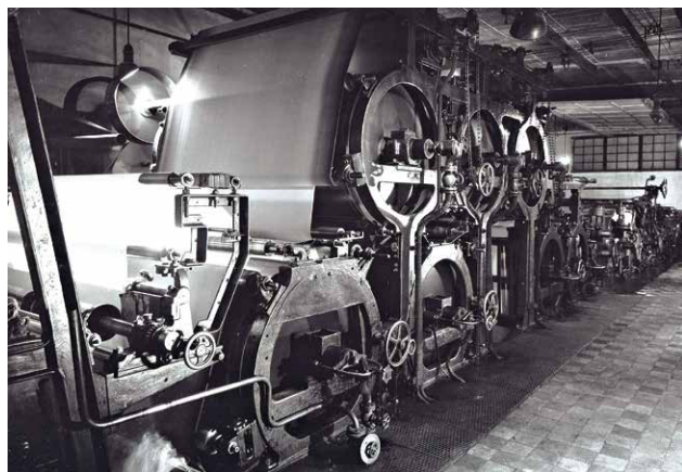
Papírenský stroj I. z roku 1839. Zdroj: SOkA Praha-venkov
